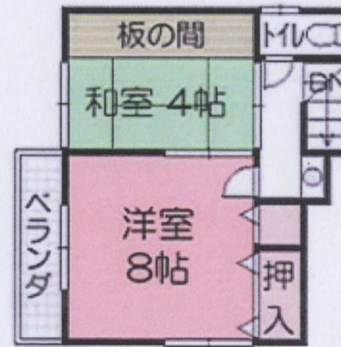
2階間取図
