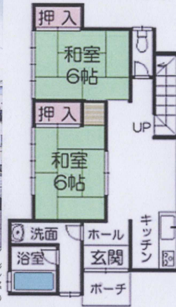
1階間取図
