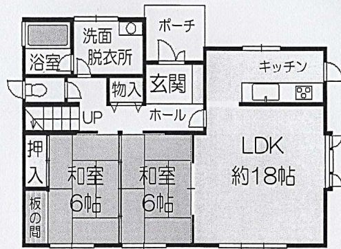
1階間取図
